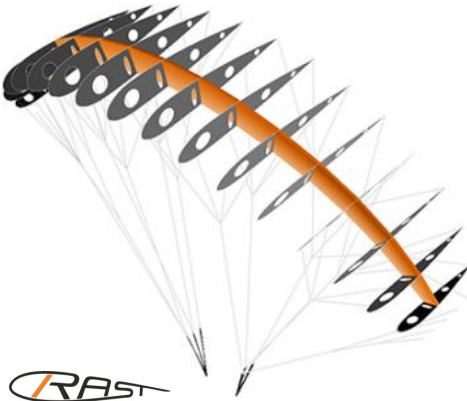
Abbildung 4 Modellzeichnung RAST
