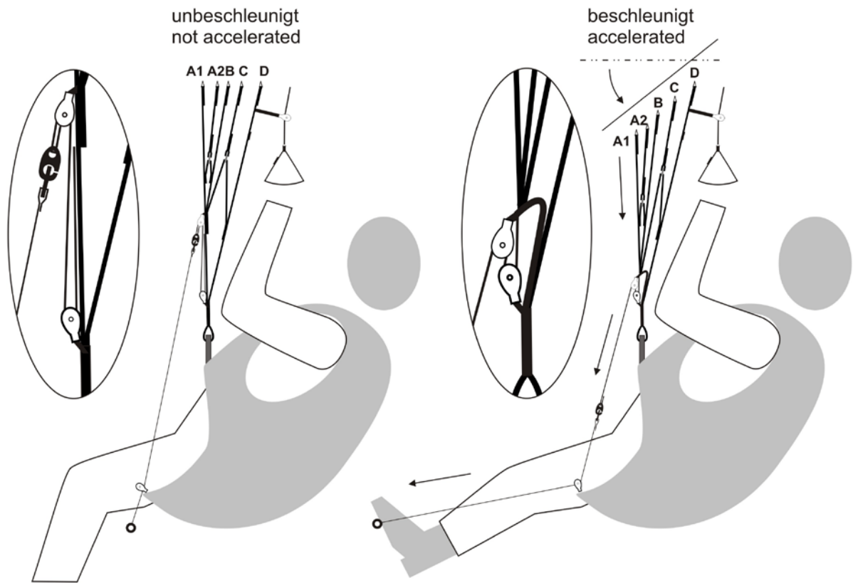
Figure 2: Comment le système d'accélérateur de l'ASTRAL 6 fonctionne
