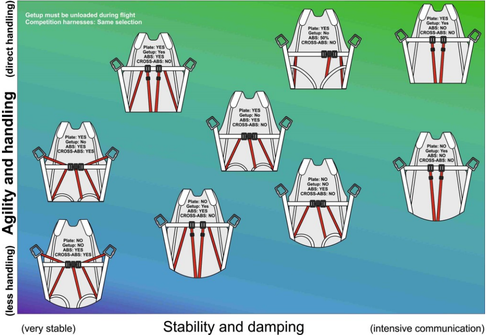
Abb. 12. Übersicht verschiedene Gurtzeuggeometrien und deren Dämpfung
