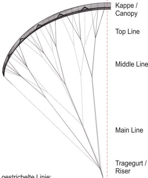
Abbildung 1: Gittermodell Twin 5
