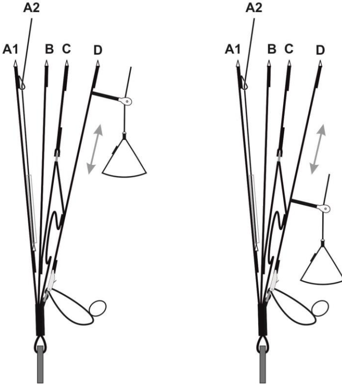
Abbildung 5: Skizze Tragegurte TWIN 5 mit Darstellung Funktionsweise Bremsslider
