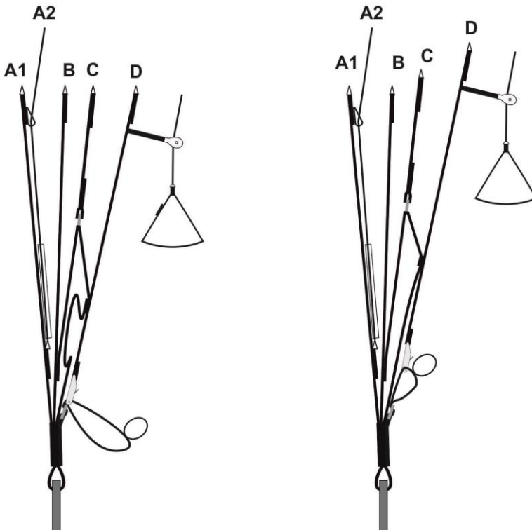
Abbildung 6: Skizze Tragegurte TWIN 5 mit Darstellung Funktionsweise Trimmer
