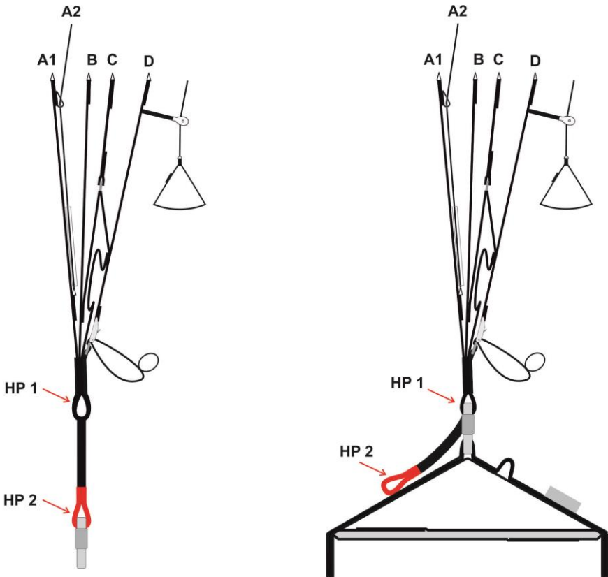
Abbildung 7: Skizze TWIN 5 S Vario Tragegurt
