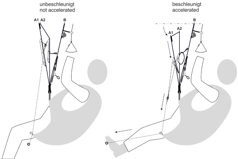
Abbildung 5: Funktionsweise Fußbeschleuniger Core 2
