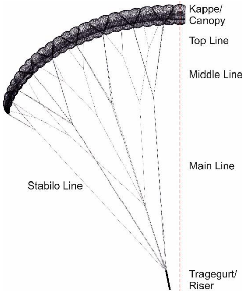
Abbildung 1: Gittermodell Nyos
