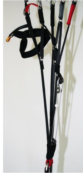
Fig. 3 NYOS RS riser
