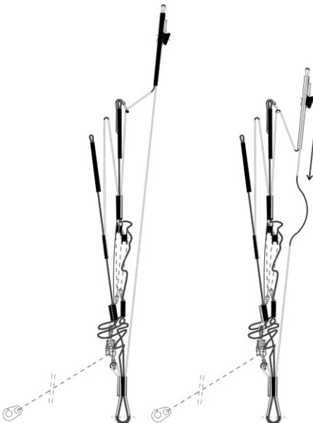
Abb. 5. Stabilisierung mit C-Stege
