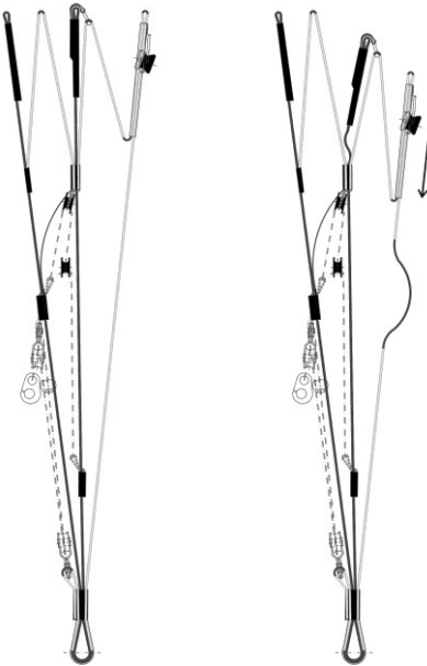
Abb. 4. Korrektur mit C-Stege
