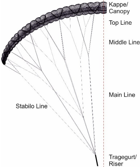
Abb. 1. Gittermodell NYOS 2 RS
