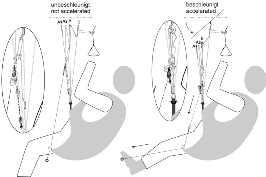
Abb. 3. Funktionsweise Fußbeschleuniger NYOS 2 RS
