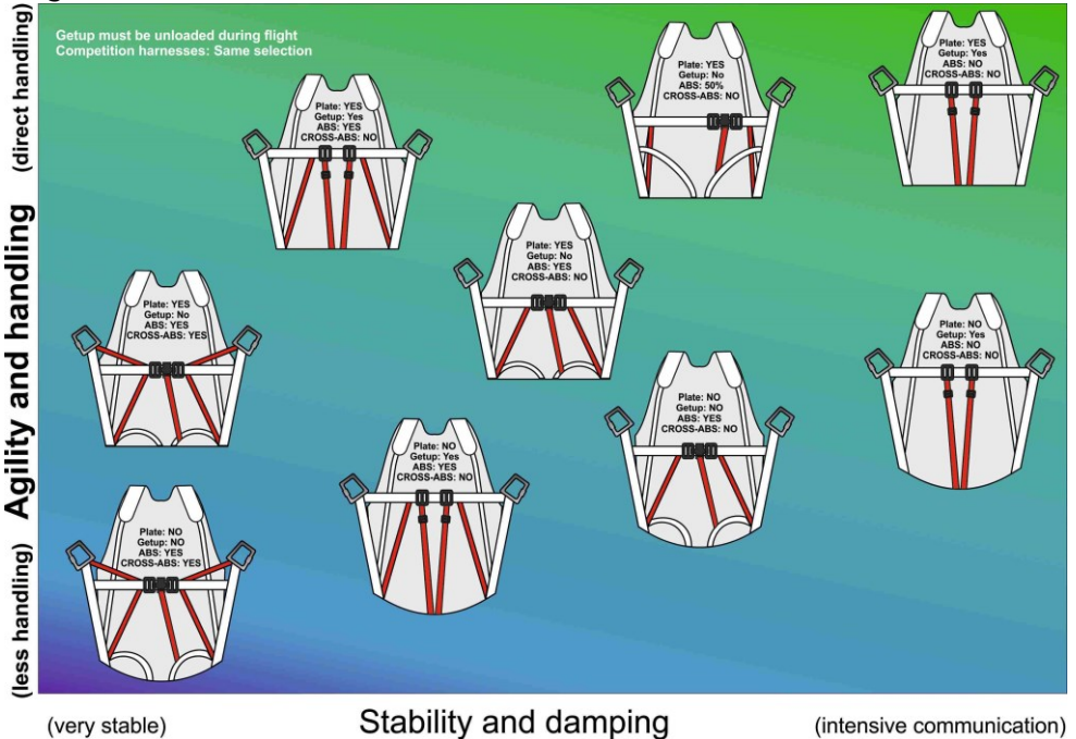
Abb. 6. Übersicht verschiedene Gurtzeuggeometrien und deren Dämpfung
