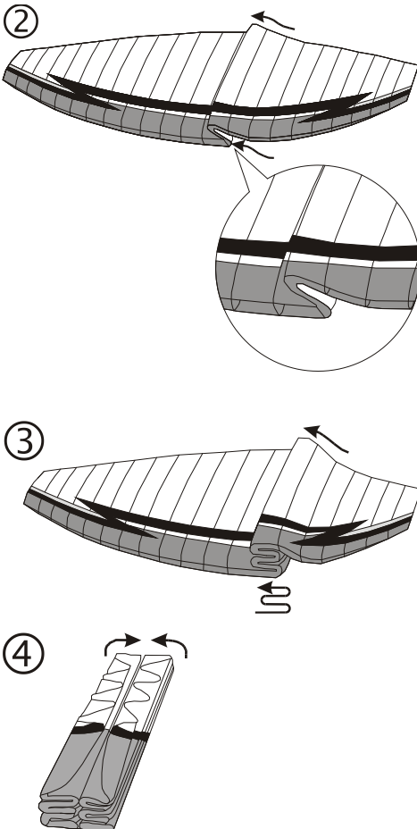
Abb. 7. Bildfolge Zusammenlegen des NYOS 2 RS
