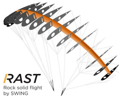
Abb. 2. Modellzeichnung RAST
