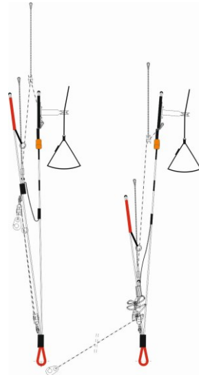
Abb. 3. Tragegurt LIBRA RS
