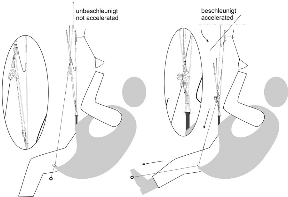
Abb. 6. Funktionsweise Fußbeschleuniger LIBRA RS
