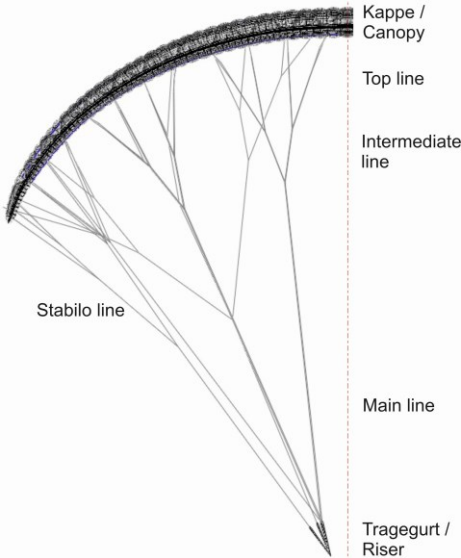
Abb. 1. Gittermodell LIBRA RS
