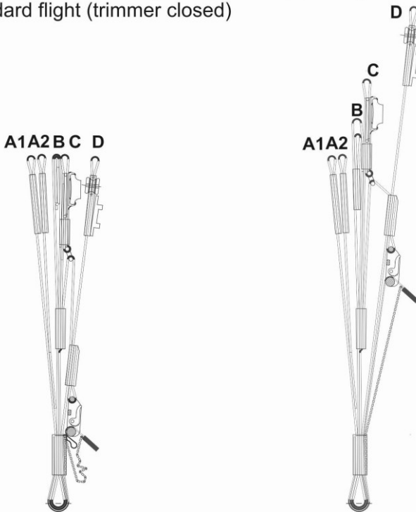
Abbildung 7: Skizze der Tragegurte TWIN 3 RS mit Darstellung der Funktionsweise des Trimmers
