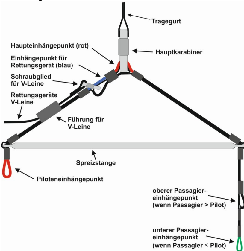
Abbildung 9: Doppelsitzerwaage
