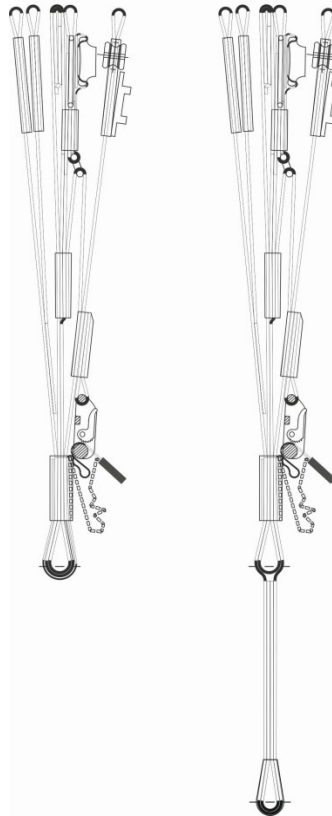
Abbildung 3: Tragegurte TWIN 3 RS
