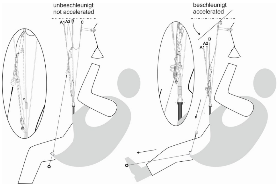
Abb. 6. Funktionsweise Fußbeschleuniger VERSO RS
