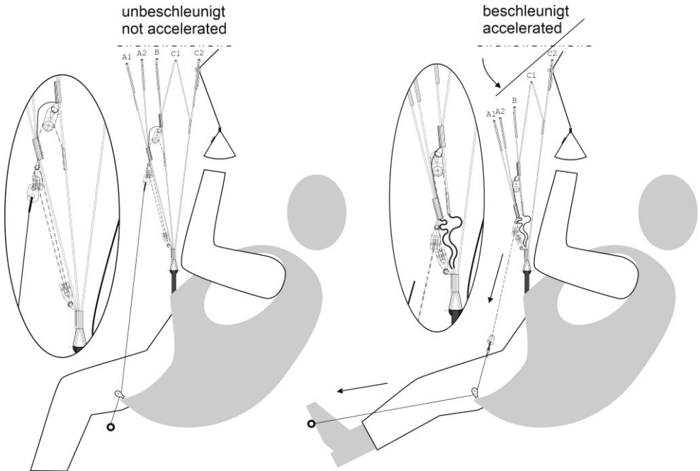
Fig. 6 Funktionsweise Fußbeschleuniger MITO 3 RS
