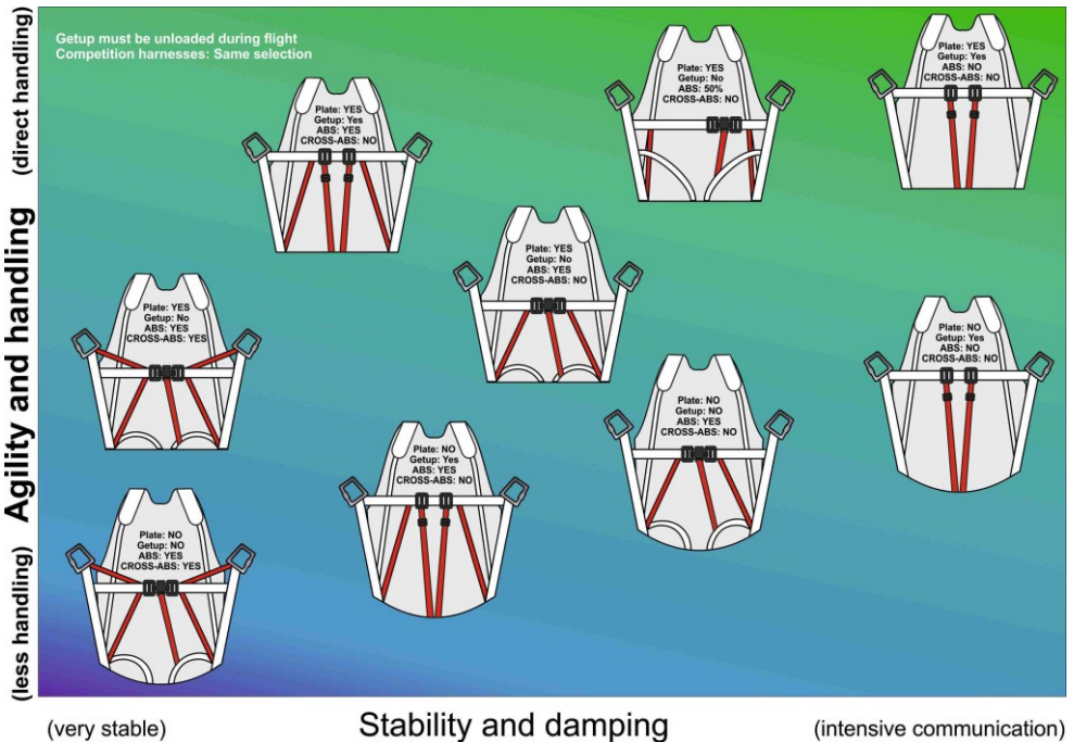
Fig. 8 Übersicht verschiedene Gurtzeuggeometrien und deren Dämpfung
