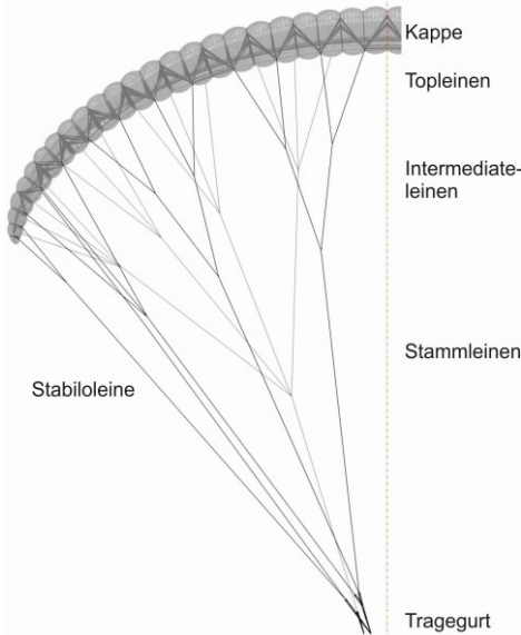
Fig. 1 Gittermodell MITO 3 RS
